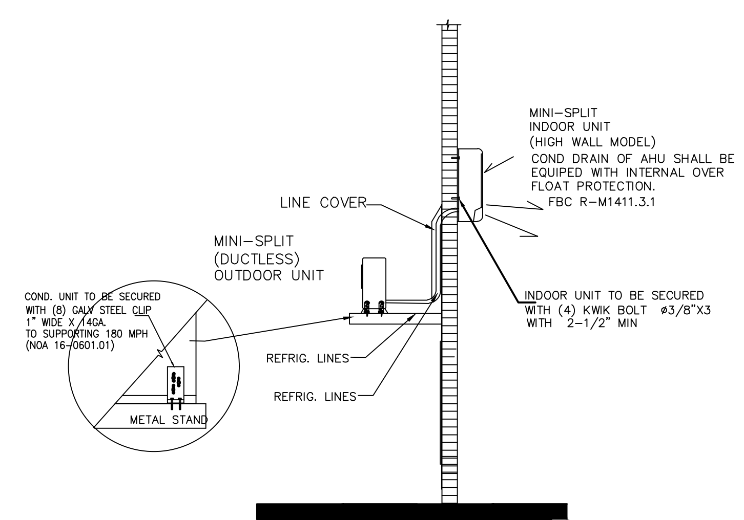
MINI-SPLIT -WALL MOUNTING DET. SCALE: N.T.S.
